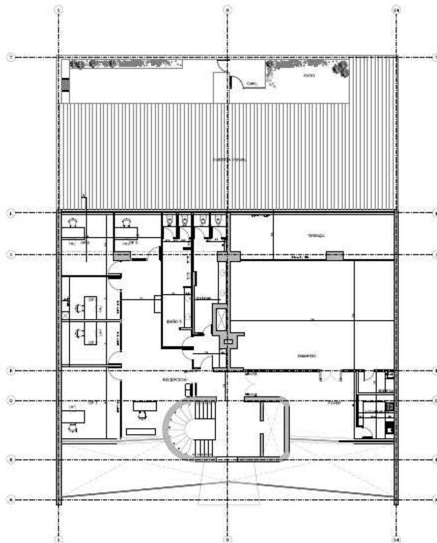
PLANTA NIVEL 2 ESC 1:100
