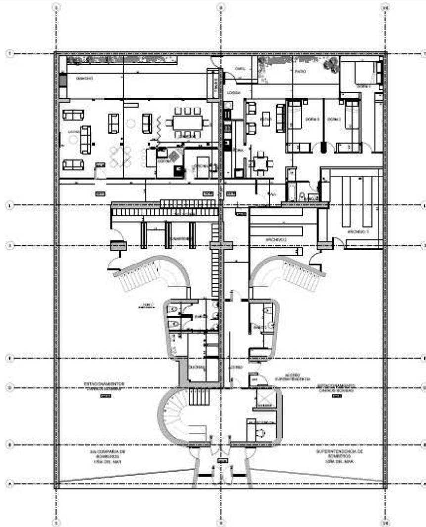
PLANTA NIVEL 1 ESC 1:100
