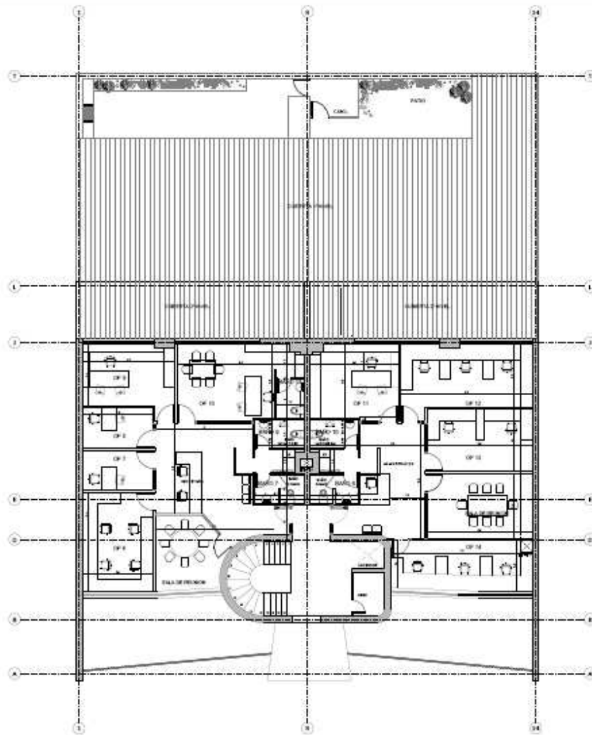
PLANTA NIVEL 3 ESC 1:100
